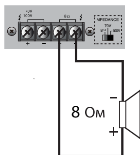
Подключение к 8 Ом
